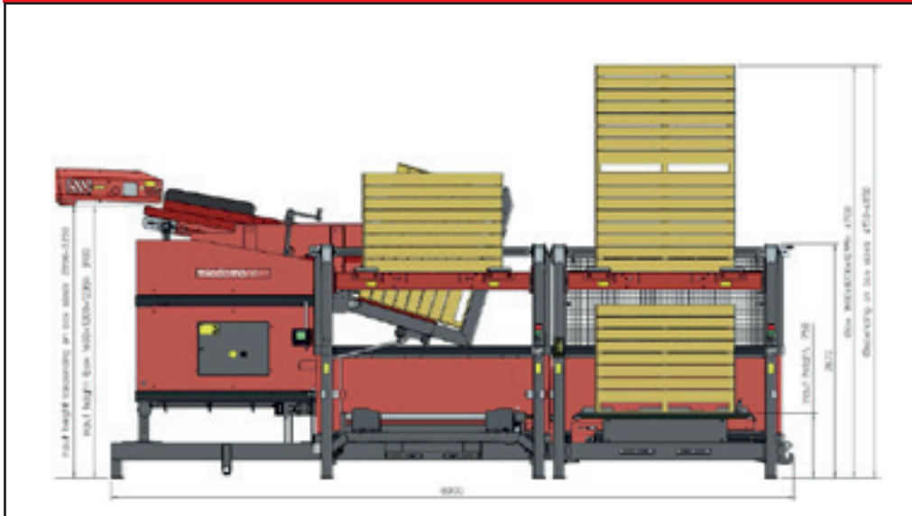
MIEDEMA MB 111
